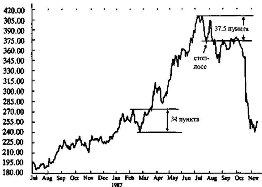
Рисунок 64 Замыкающий стоп-лосс.
